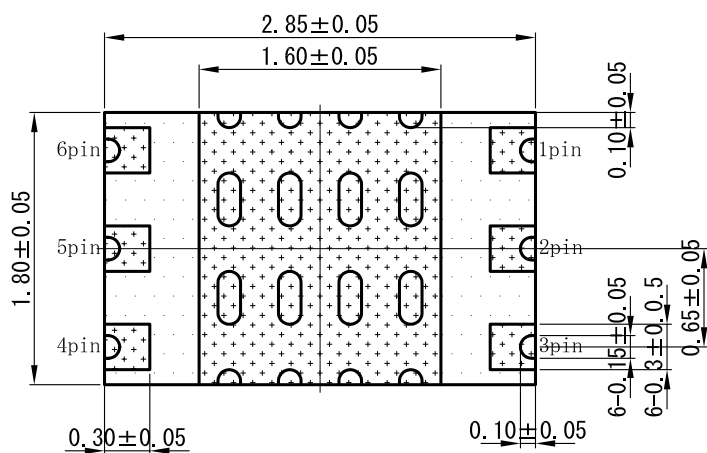
実装面
