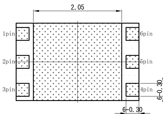
インナーリード部図
