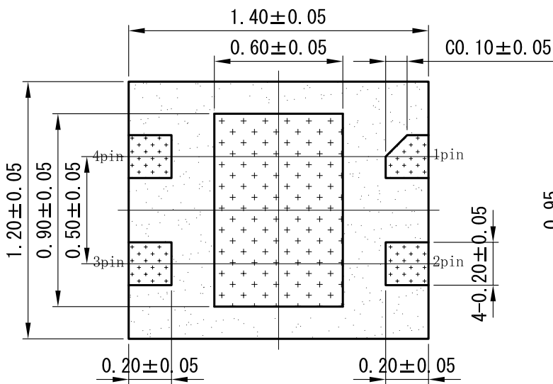
実装面
