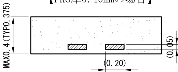
【PKG厚0.40mmの場合】
