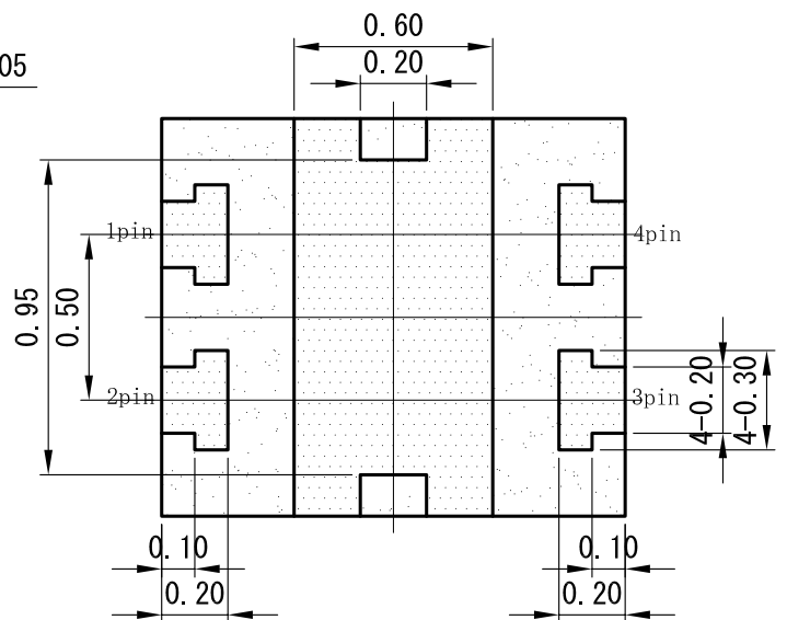
インナーリード部
